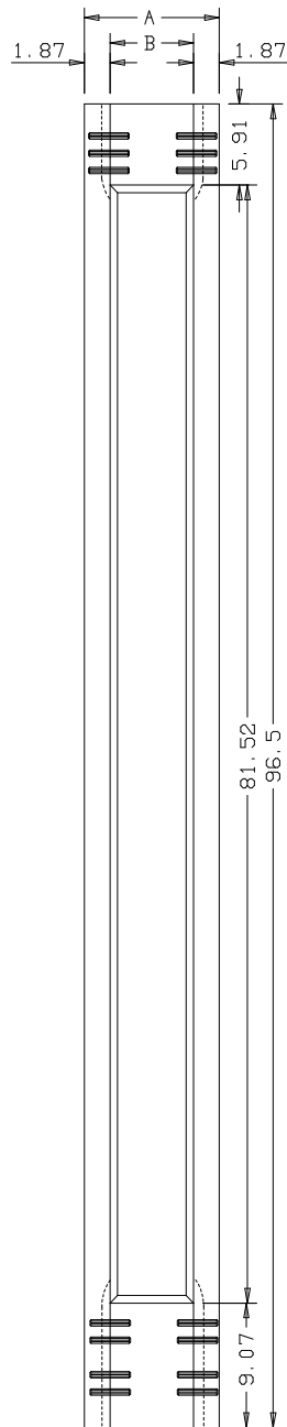
Ovolo Sticking
